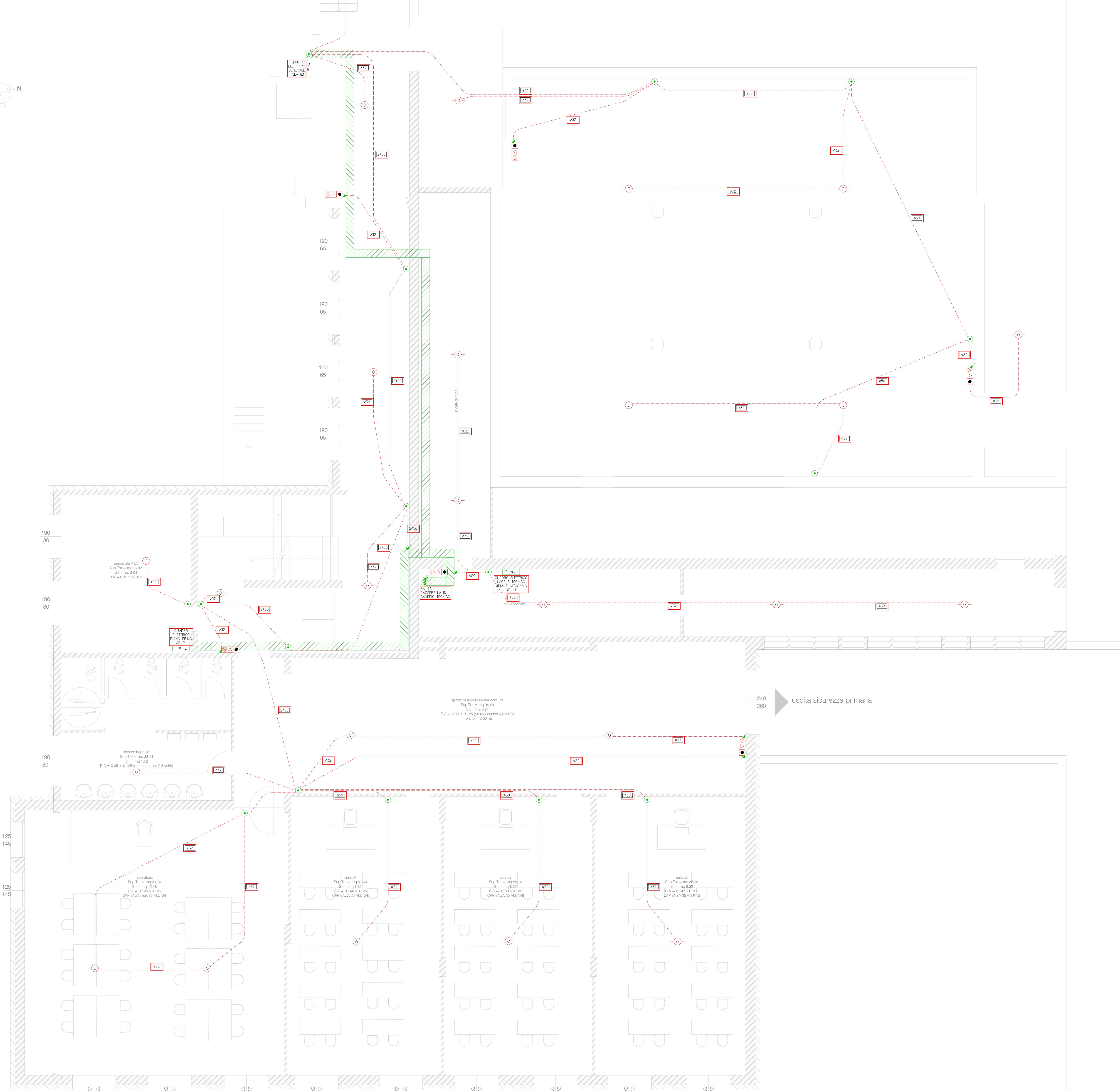
Planimetria piano primo – Impianti rivelazione fumi – scala 1:50
